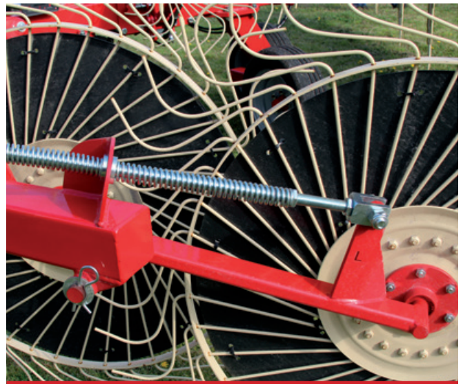
Bracci per ruote stellari indipendenti. / Independent rake wheel arms. / Brazos de soles independientes. / Système ressorts des bras.
